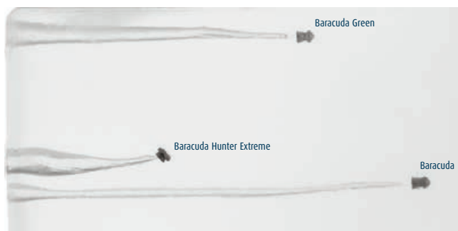
Test mit ballistischer Seife / Test with ballistic soap / Βαλιστικός έλεγχος
